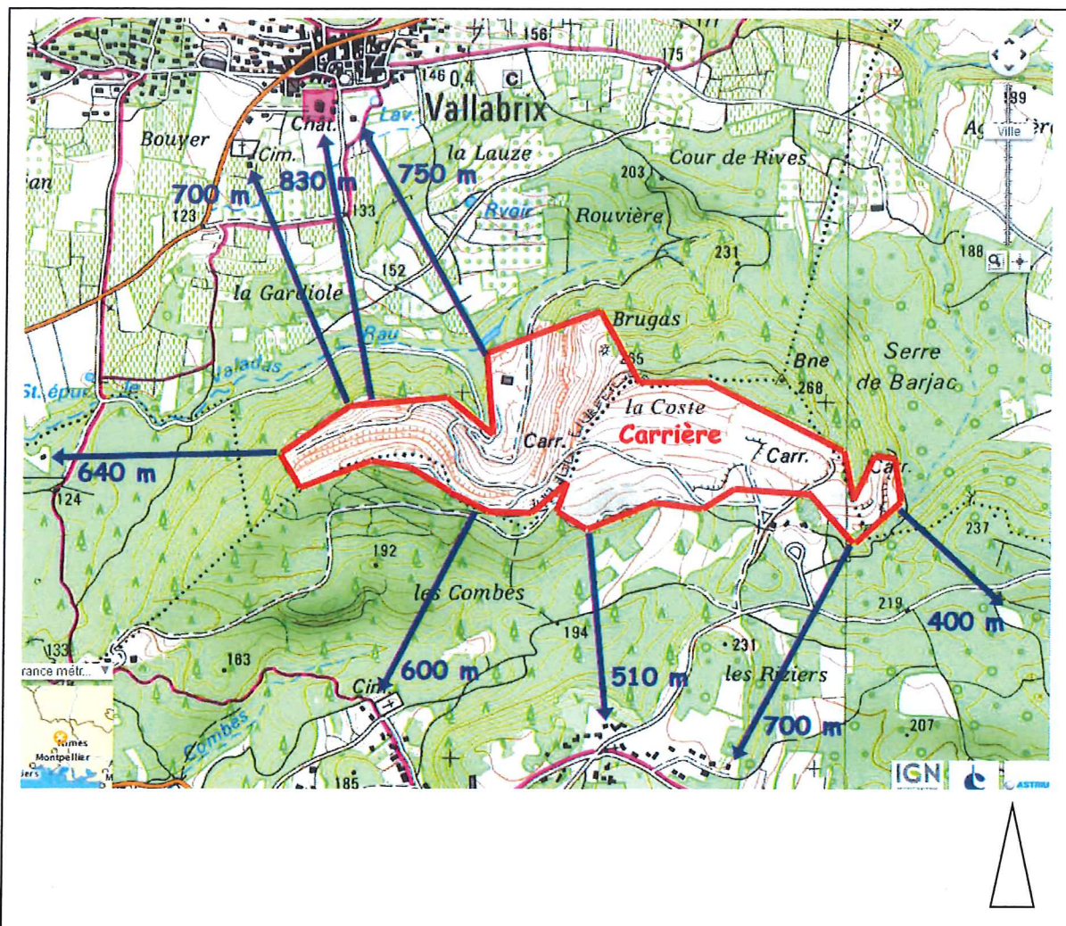
CARRIÈRE DE VALLABRIX (30) : DISTANCES ENTRE LA CARRIÈRE ET LES PRINCIPALES HABITATIONS
